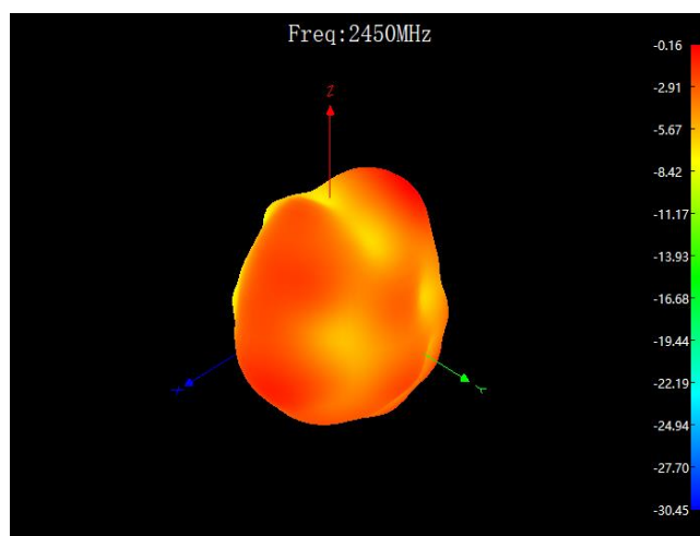
2450MHz 3D
