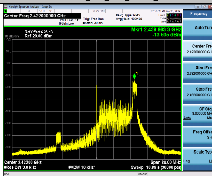
11AX40SISO_Ant1_2422_52Tone_RU37
