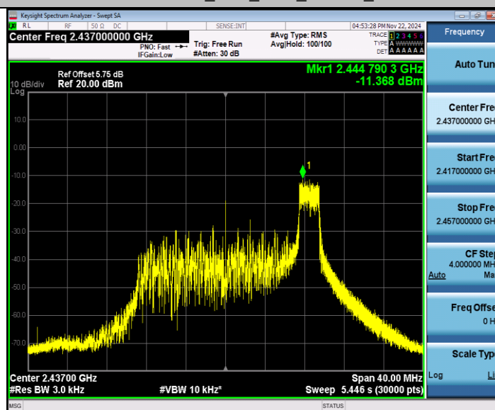
11AX20SISO_Ant1_2437_52Tone_RU37
