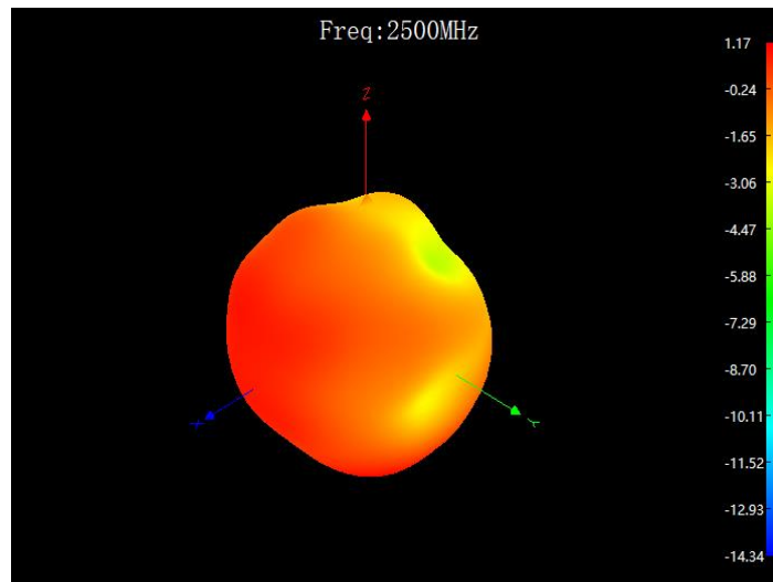
2500MHz 3D
