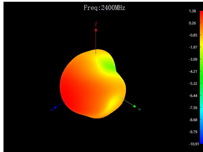
2450MHz 3D
