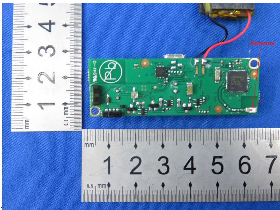
EUT Antenna:
