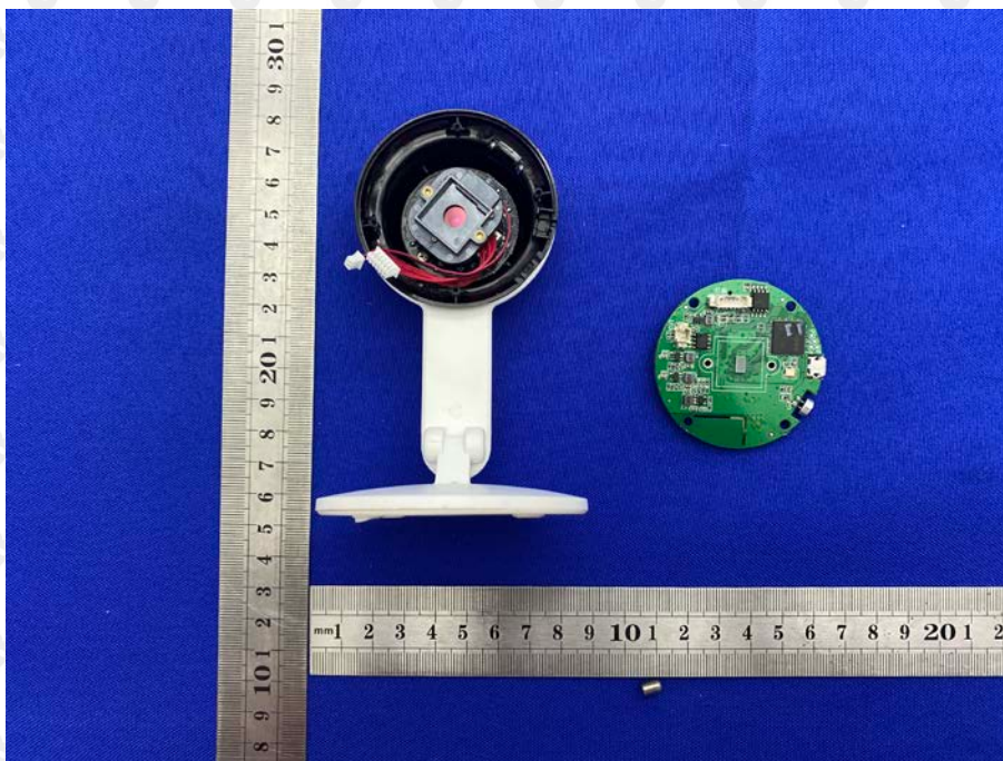
EUT Photo 9
