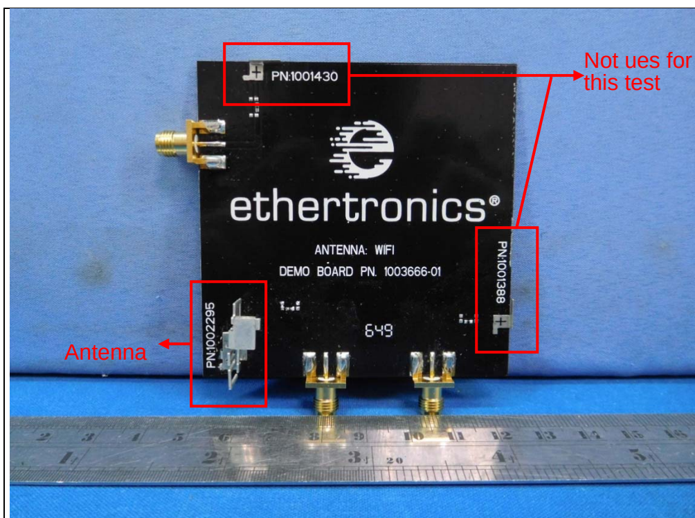
Antenna set 4
