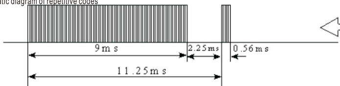
发码数据参数示意图 Sketch map of hair code
