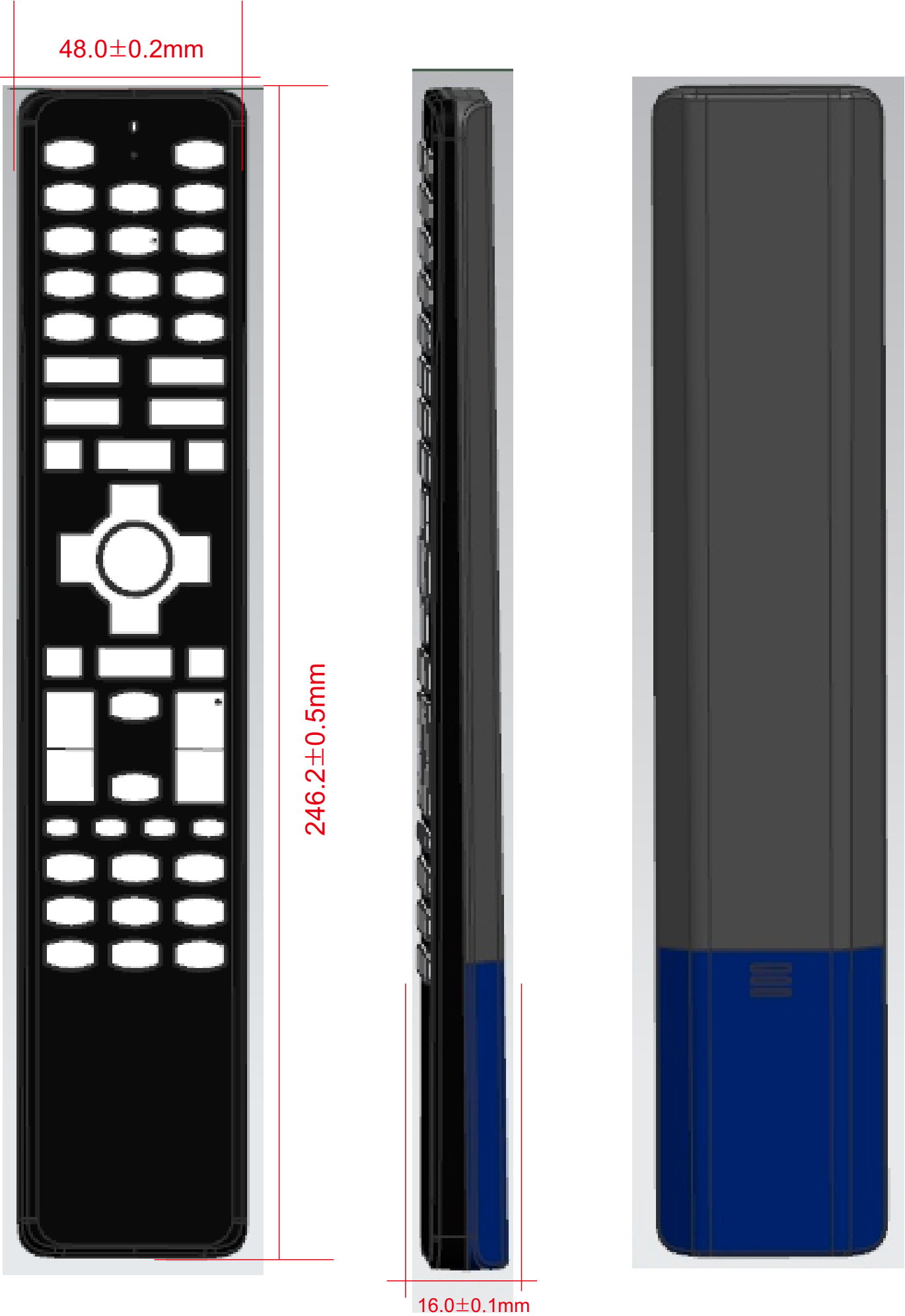
五. 外观尺寸图/DIMENSIONS FIG
