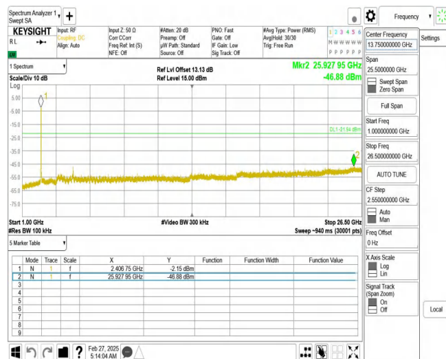
11G_Ant1_2412_1000~26500
