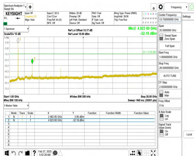
11B_Ant1_2462_1000~26500
