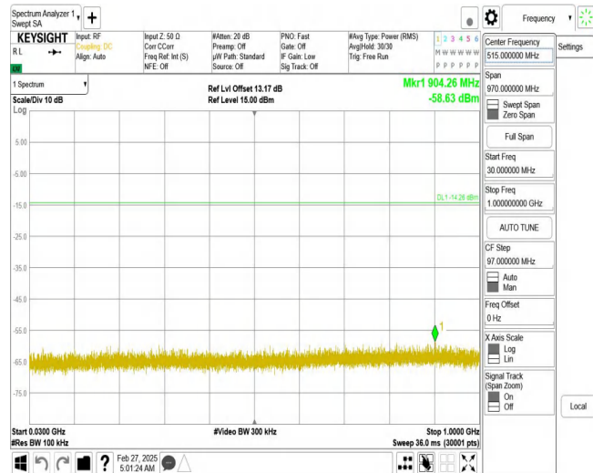
11B_Ant1_2462_30~1000
