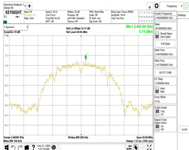
11B_Ant1_2462_0~Reference
