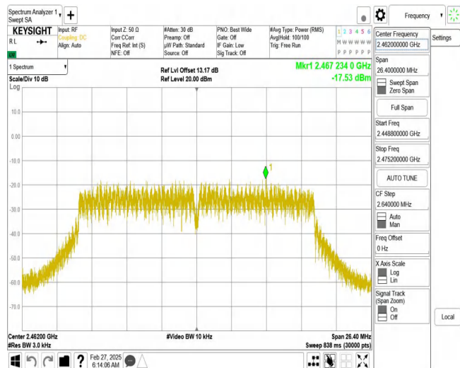
11N20SISO_Ant1_2462
