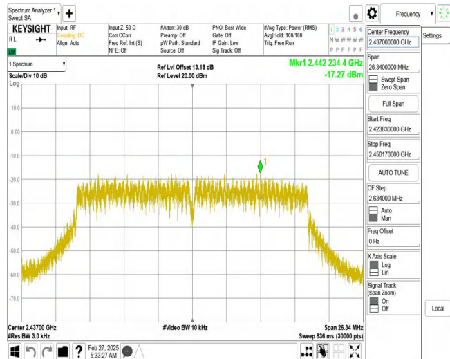
11N20SISO_Ant1_2437
