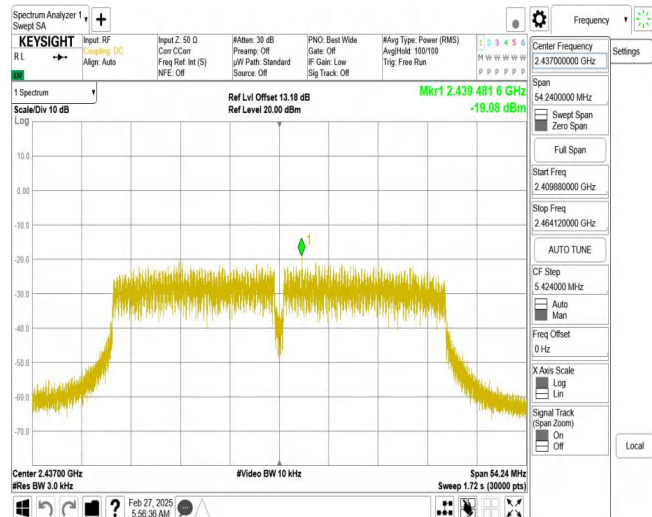
11N40SISO_Ant1_2437
