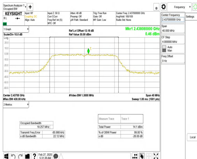
11N20SISO_Ant1_2437
