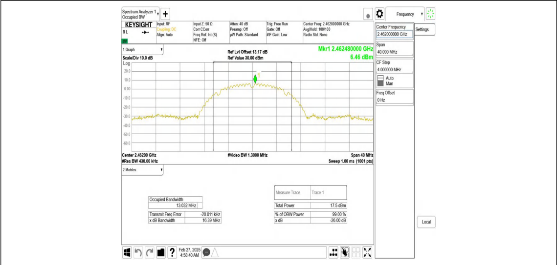
11B_Ant1_2462
