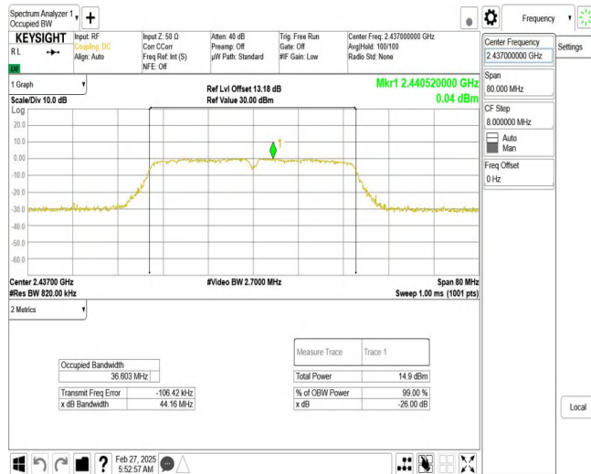
11N40SISO_Ant1_2437
