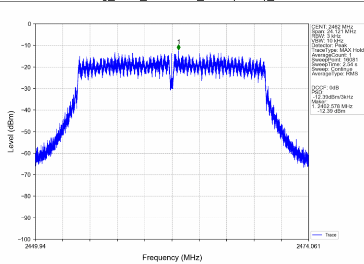
802.11g_HCH_2462MHz_Ant1 (SISO)_NTNV
