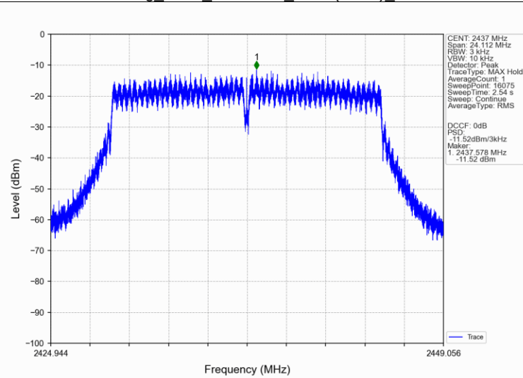
802.11g_MCH_2437MHz_Ant1 (SISO)_NTNV
