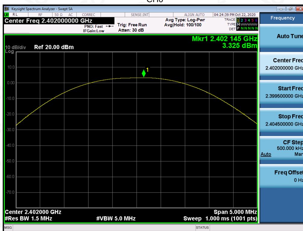
\text{CHO}
