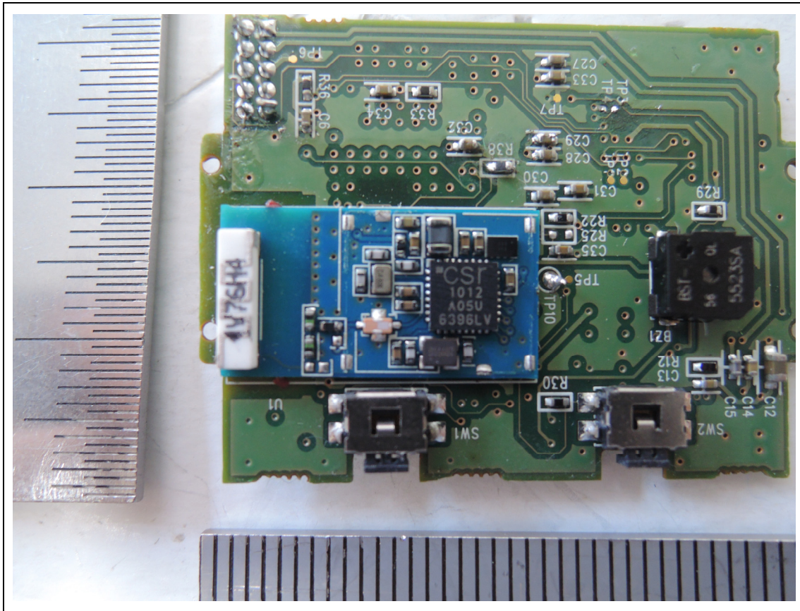
&lt;Module&gt;
