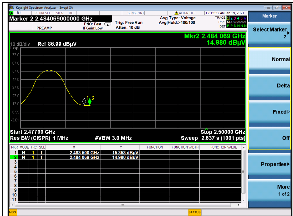
(AVERAGE, Channel 26)
