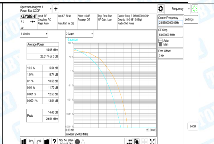
41(2535-2655)-20MHz-16QAM-40590-100RB#0-PASS
