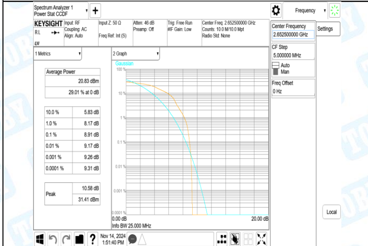
41(2535-2655)-10MHz-QPSK-40090-1RB#0-PASS
