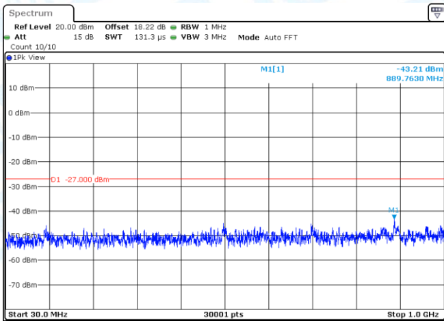
11AC80SISO-Ant1-5290-30~1000-PASS
