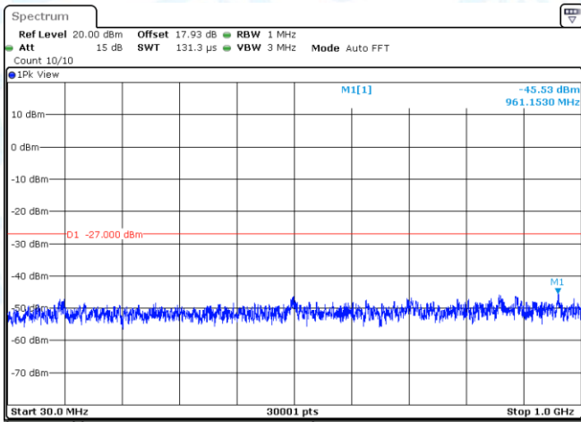
11AC80SISO-Ant1-5210-30~1000-PASS
