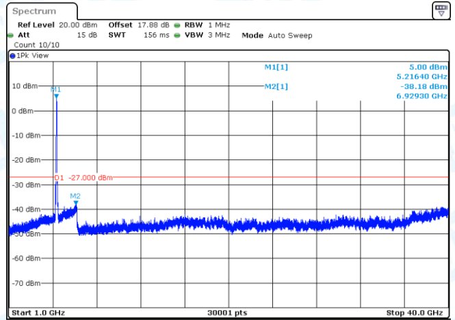
11AC80SISO-Ant1-5210-1000~40000-PASS
