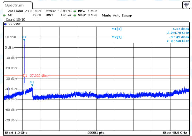
11AC80SISO-Ant1-5210-1000~40000-PASS
