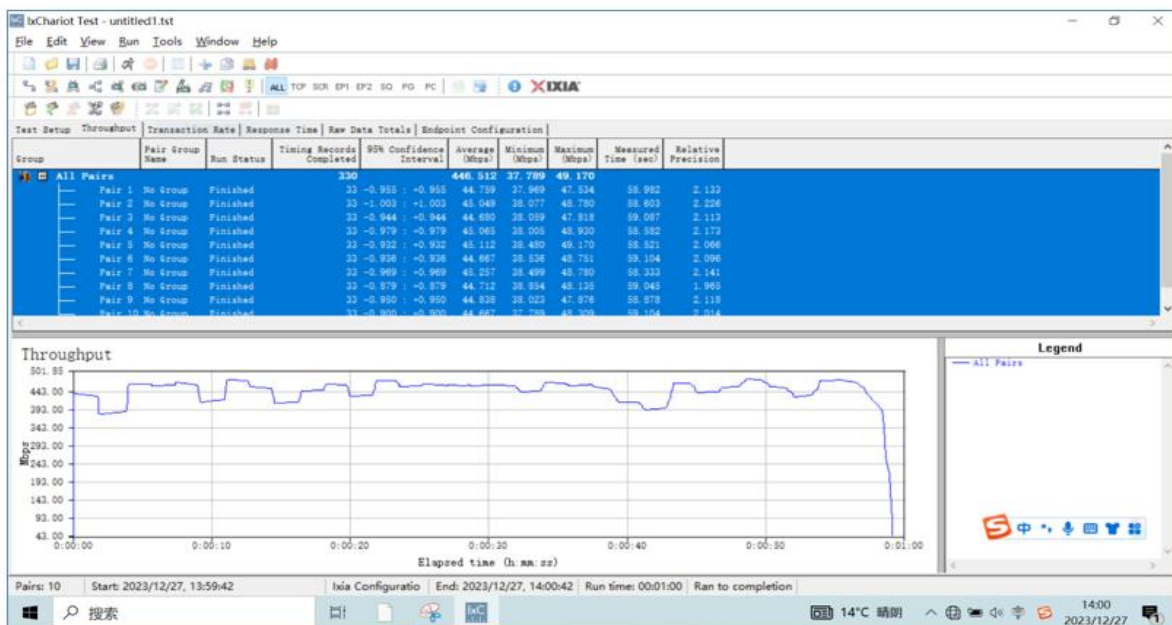
AX101 WiFi模块吞吐量发射数据
