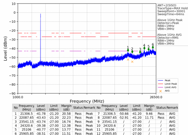
802.11a_LCH_5180MHz_Ant2_NTNV
