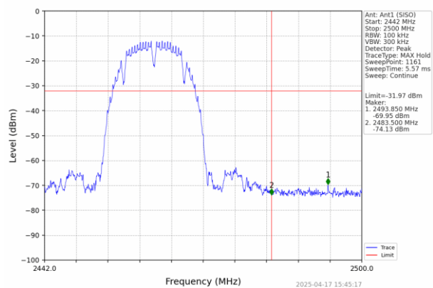
802.11b_HCH_2462MHz_Ant1 (SISO)_NTNV
