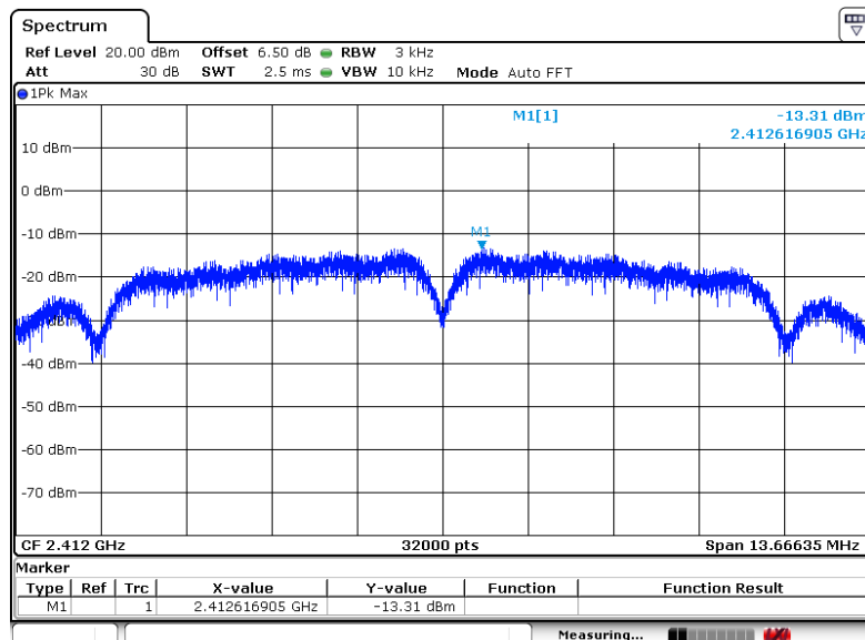
802.11 B Mode CH1
