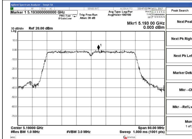
Chain 0-802.11n40-5190MHz
