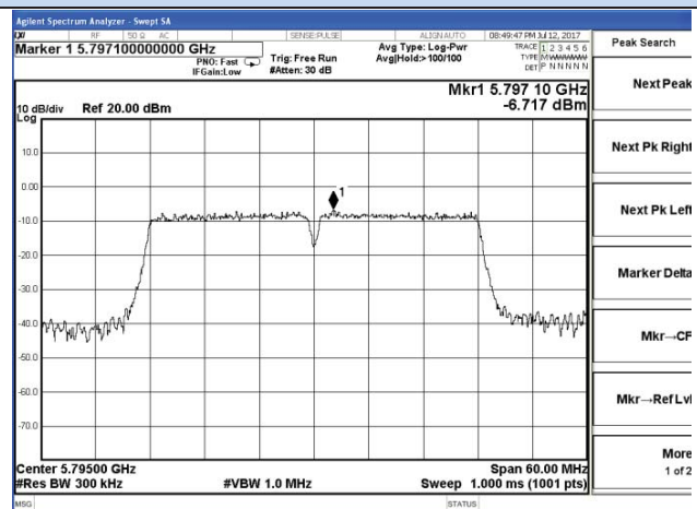
Chain 1-802.11n40-5795MHz
