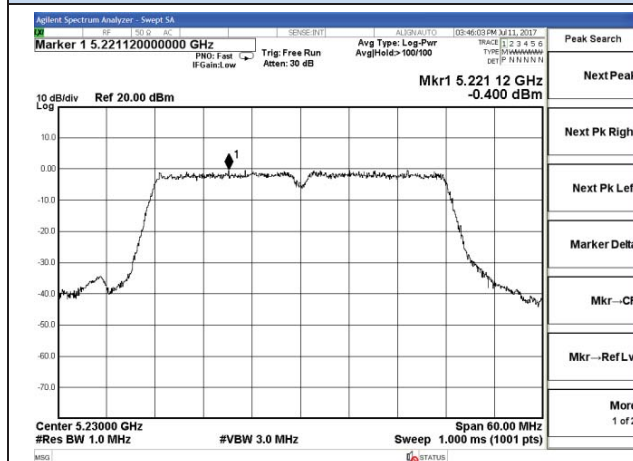
Chain 0-802.11n40-5230MHz
