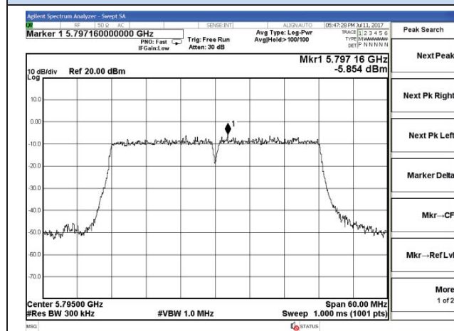
Chain 0-802.11n40-5795MHz
