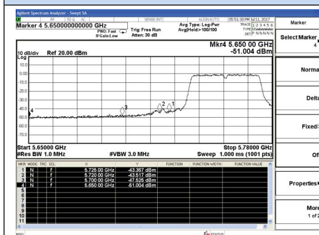
802.11n40-5755MHz-Lower
