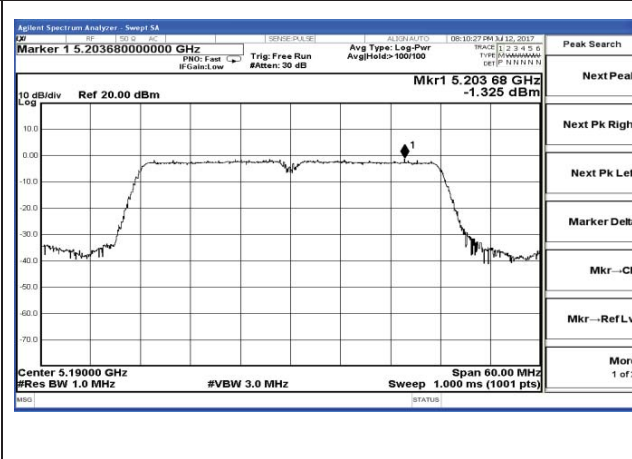
Chain 1-802.11n40-5190MHz
