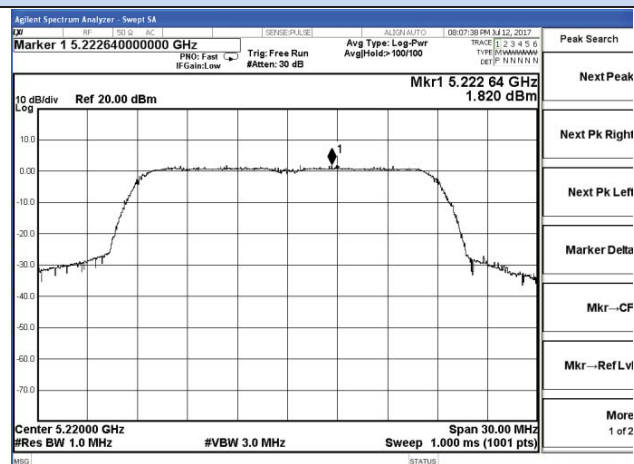
Chain 1-802.11n20-5220MHz
