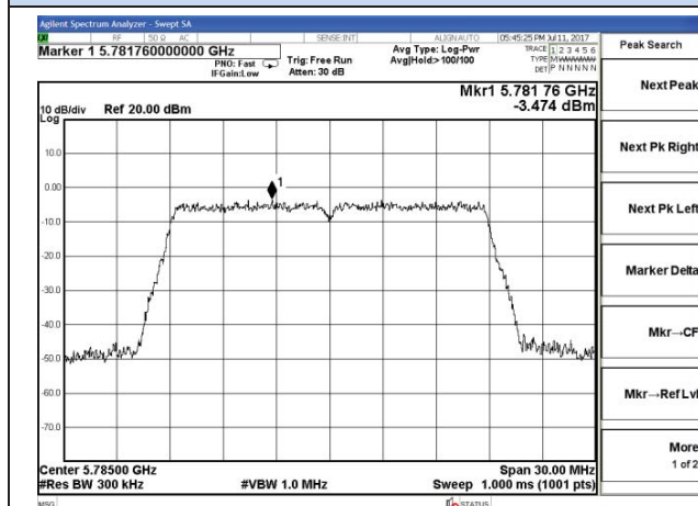
Chain 0-802.11n20-5785MHz
