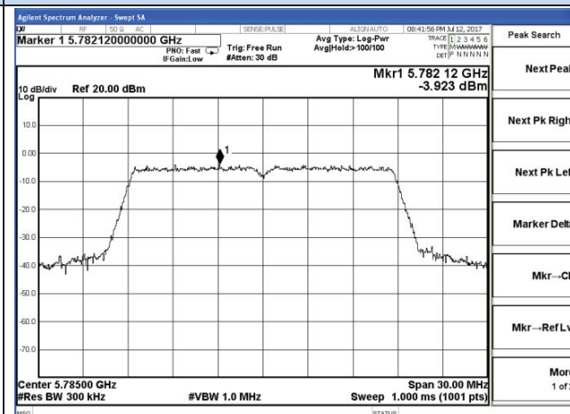
Chain 1-802.11n20-5785MHz
