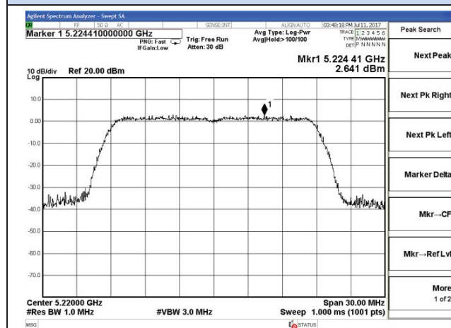
Chain 0-802.11n20-5220MHz
