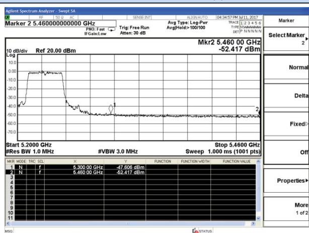
802.11n40-5230MHz-Upper
