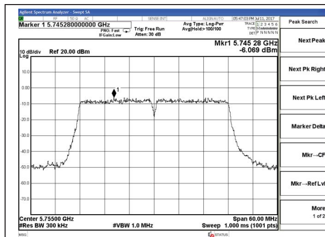
Chain 0-802.11n40-5755MHz
