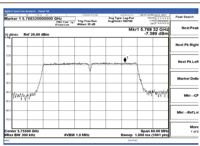
Chain 1-802.11n40-5755MHz
