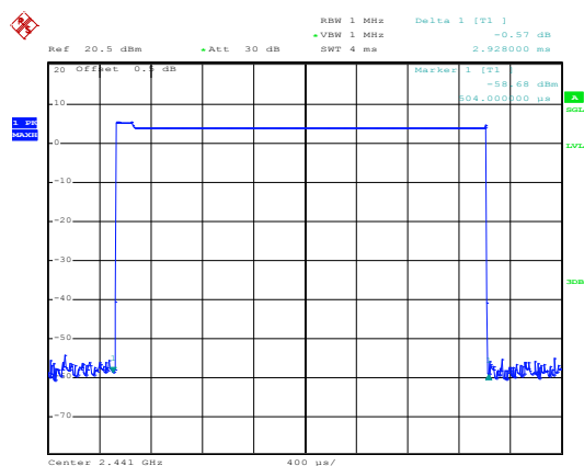
2-DH5
