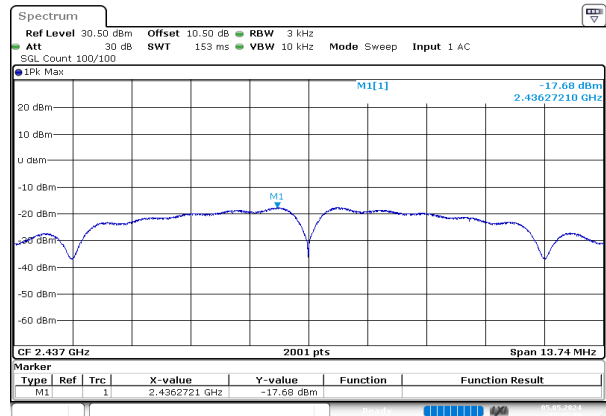
b_2437MHz_Chain 0
