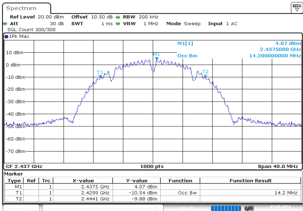
b_2437MHz_Chain 0
