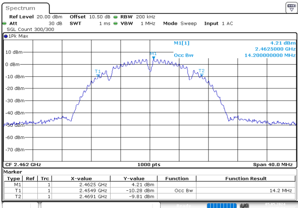
b_2462MHz_Chain 0
