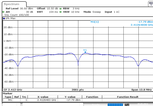
b_2412MHz_Chain 0
