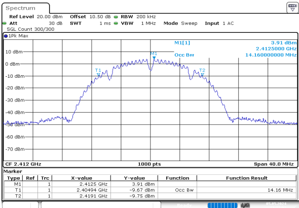
b_2412MHz_Chain 0
