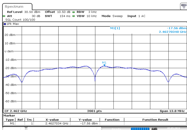
b_2462MHz_Chain 0
