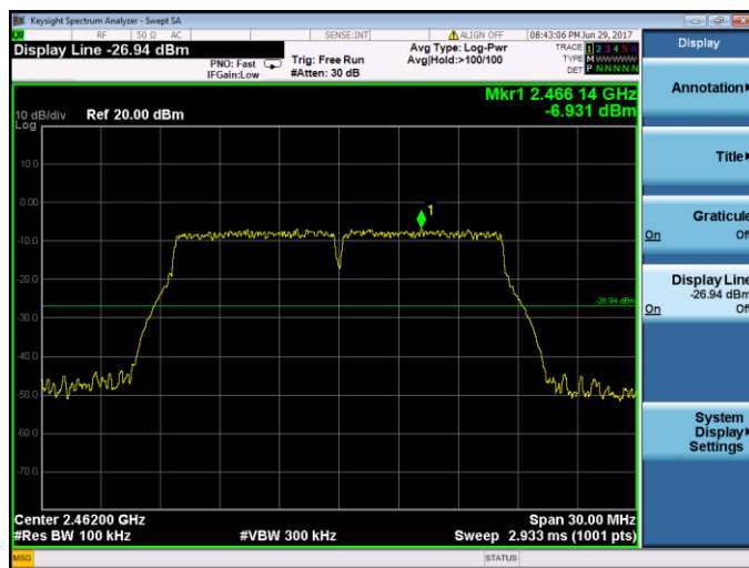
IEEE 802.11g-Channel 11 / 2462 MHz
