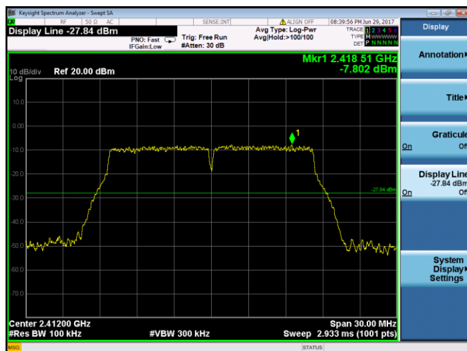
IEEE 802.11g-Channel 1 / 2412 MHz
