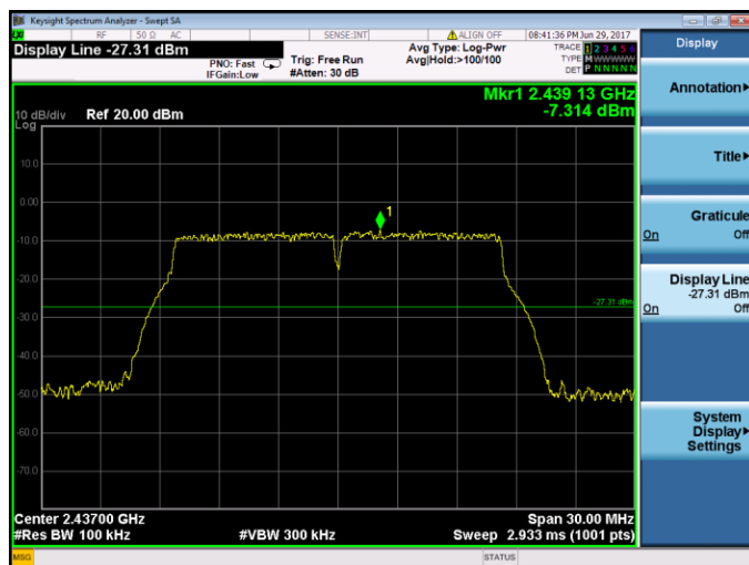
IEEE 802.11g-Channel 6 / 2437 MHz
