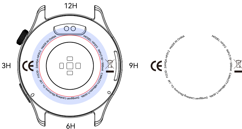
■ 镭雕内容 SCALE 1:1
