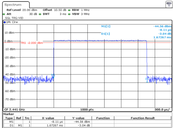
DH3_Hopping 1.673ms
