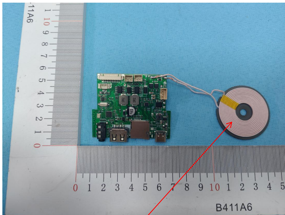
WPT-ANT
