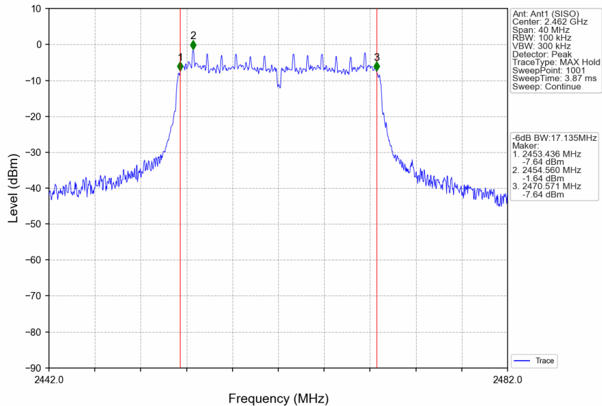
802.11n(HT20)_HCH_2462MHz_Ant1 (SISO)_NTNV
