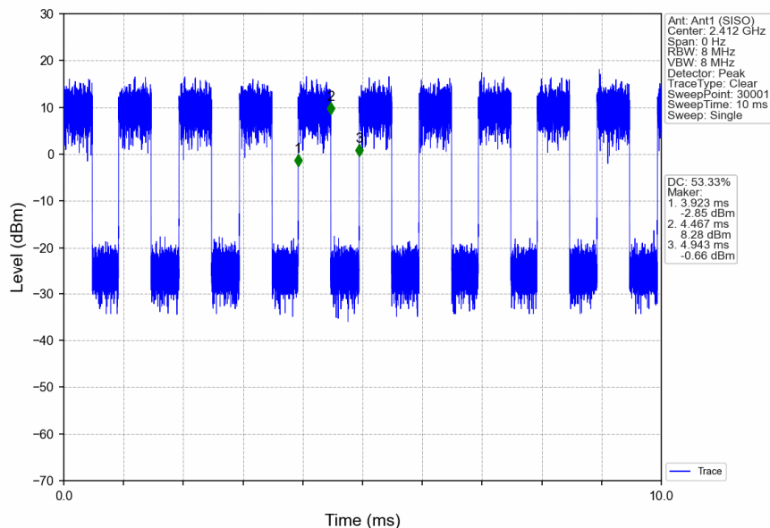
802.11g_LCH_2412MHz_Ant1 (SISO)_NTNV
