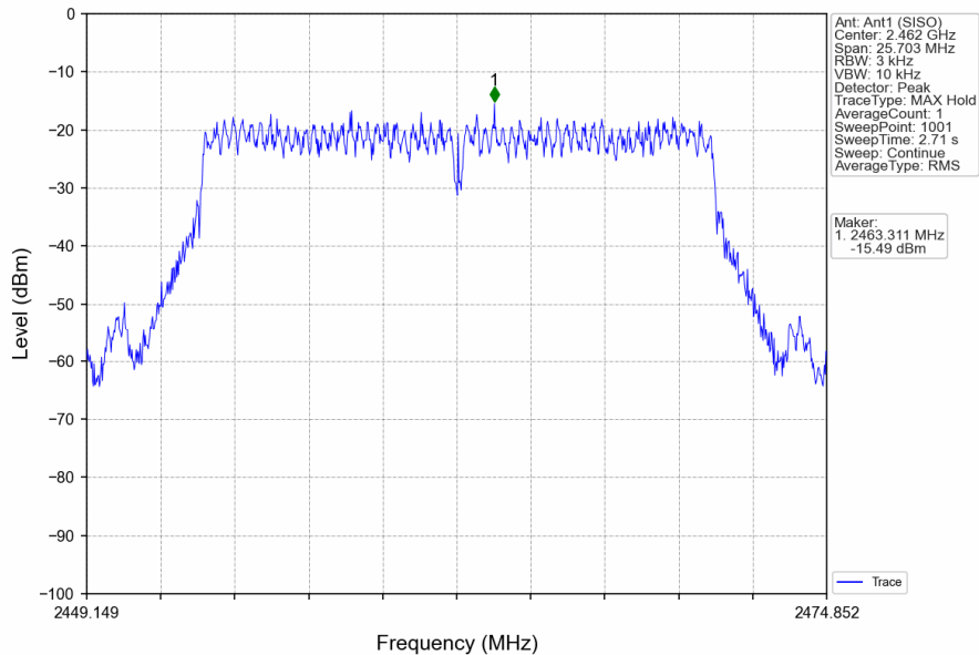
802.11n(HT20)_HCH_2462MHz_Ant1 (SISO)_NTNV
