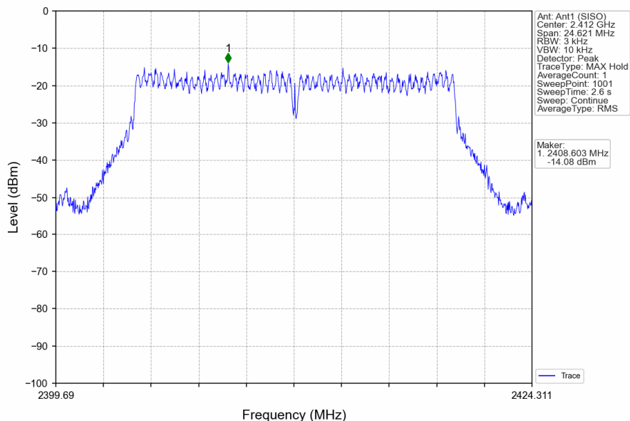
802.11g_LCH_2412MHz_Ant1 (SISO)_NTNV
