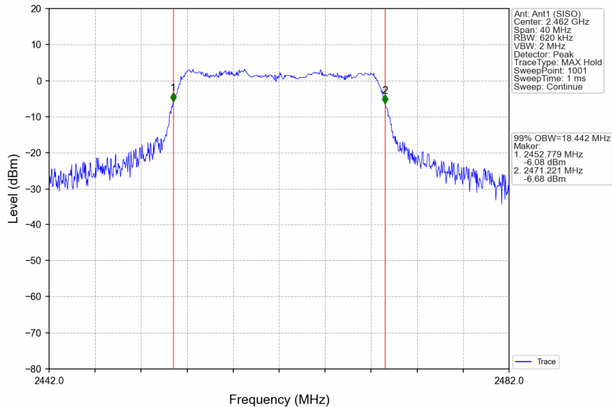
802.11n(HT20)_HCH_2462MHz_Ant1 (SISO)_NTNV
