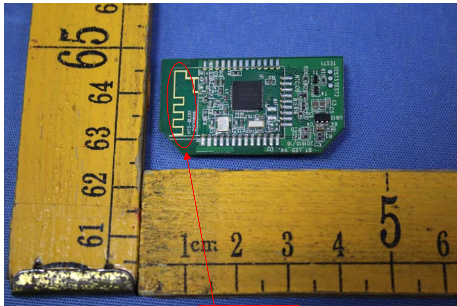
BLE ANT.
