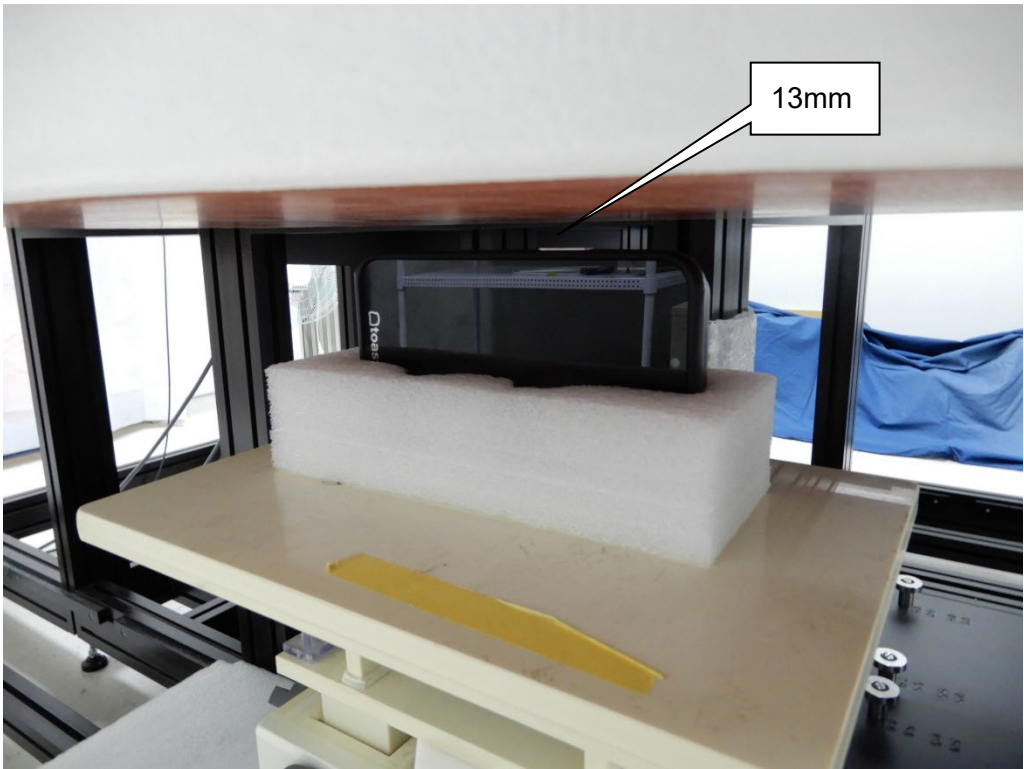
EUT Left-side_13mm
