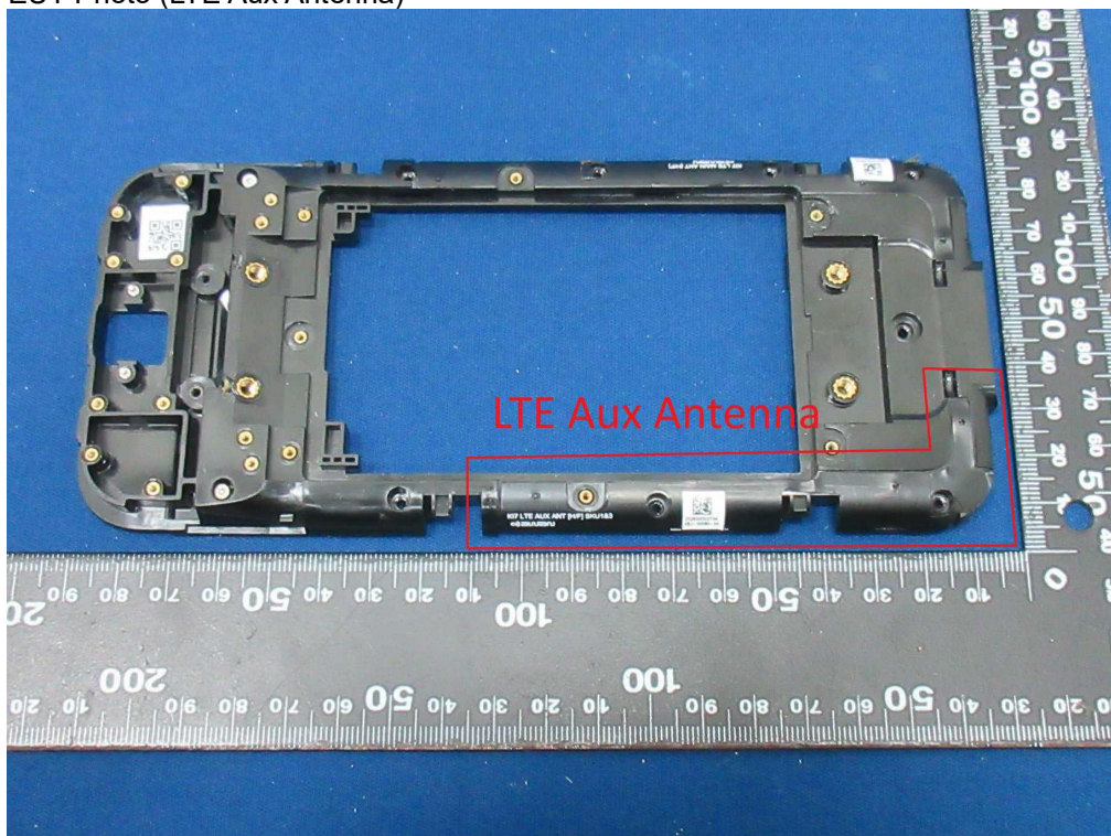
(70) EUT Photo (LTE Aux Antenna)
