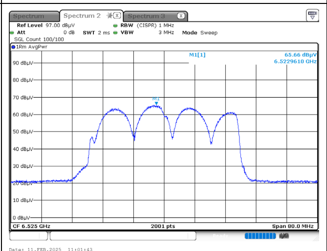
802.11ax / 40MHz / 6525MHz / Ch115
