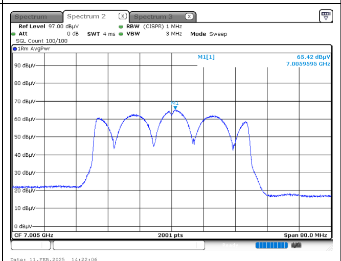
802.11ax / 40MHz / 7005MHz / Ch211
