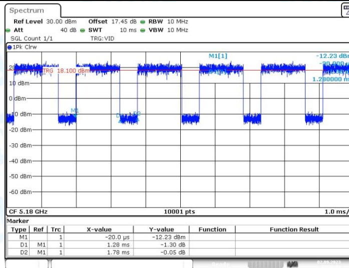
11AC20MIMO_Ant2_5180
