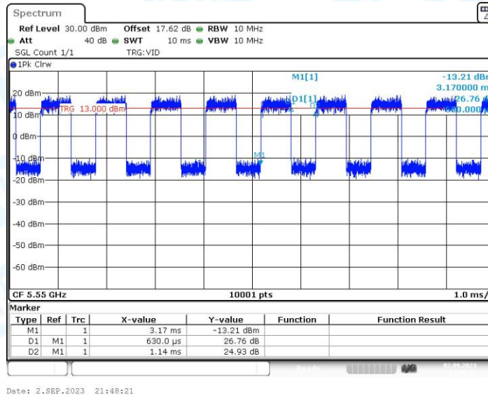
11N40MIMO_Ant2_5550
