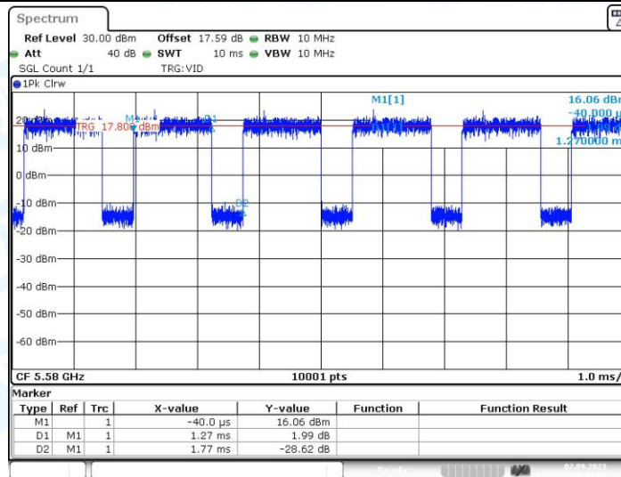
11N20MIMO_Ant1_5580
