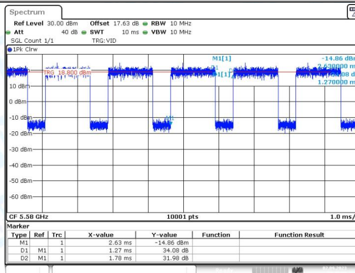
11N20MIMO_Ant2_5580
