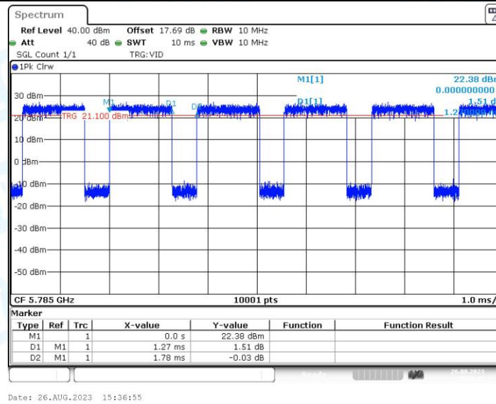
11N20MIMO_Ant2_5785
