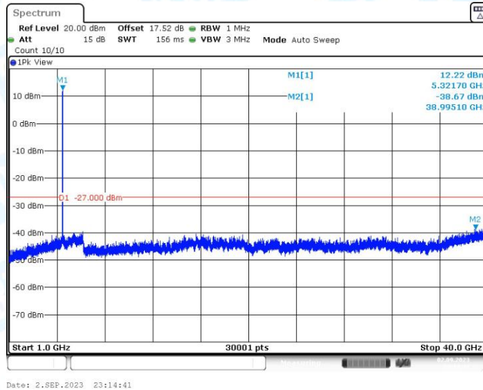
11AC20MIMO_Ant1_5500_30~1000
