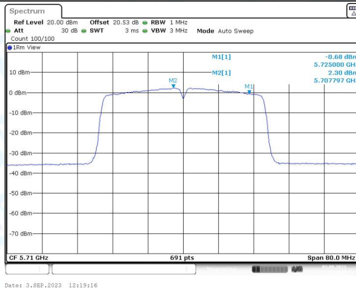
11N40MIMO_Ant1_5710_UNII-3
