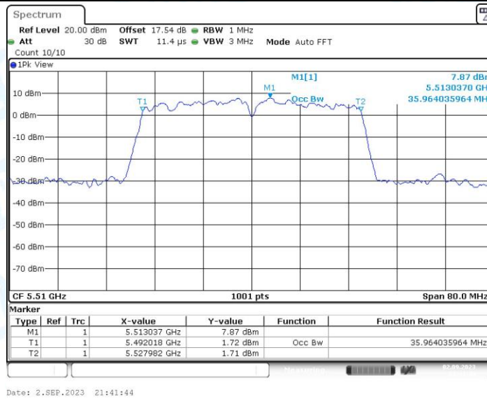
11N40MIMO_Ant2_5510
