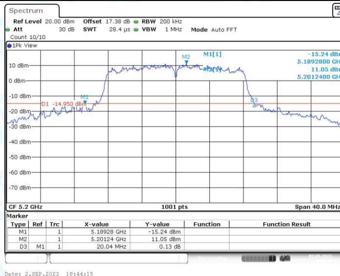
11A_Ant2_5200
