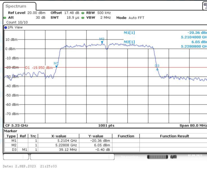
11N40MIMO_Ant2_5230
