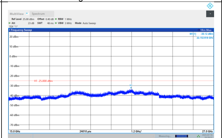
Band41-20MHz-QPSK-39750-1RB#0- Range:15000~27000MHz
