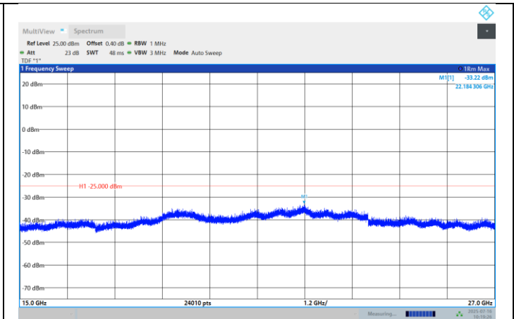
Band41-20MHz-QPSK-40620-1RB#0- Range:15000~27000MHz
