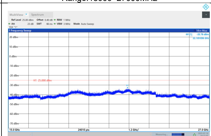
Band41-10MHz-QPSK-41540-1RB#0- Range:15000~27000MHz
