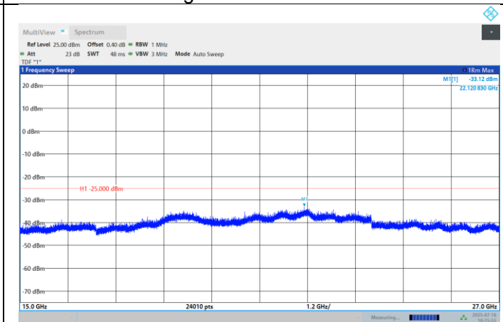
Band41-15MHz-QPSK-39725-1RB#0- Range:15000~27000MHz
