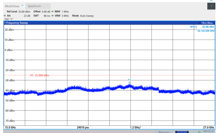
Band41-10MHz-QPSK-39700-1RB#0- Range:15000~27000MHz
