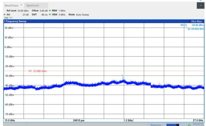
Band41-5MHz-QPSK-41565-1RB#0- Range:15000~27000MHz
