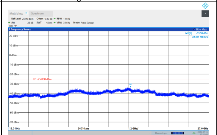
Band41-20MHz-QPSK-41490-1RB#0- Range:15000~27000MHz
