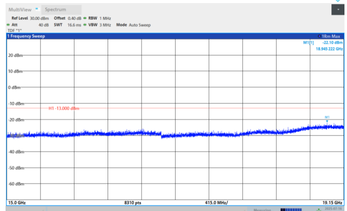
Band25-10MHz-QPSK-26340-1RB#0- Range:15000MHz~19150MHz
