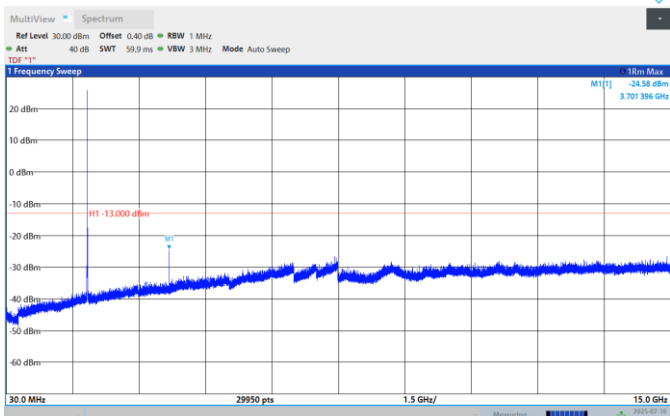
Band25-10MHz-QPSK-26340-1RB#0-Range:30~15000MHz
