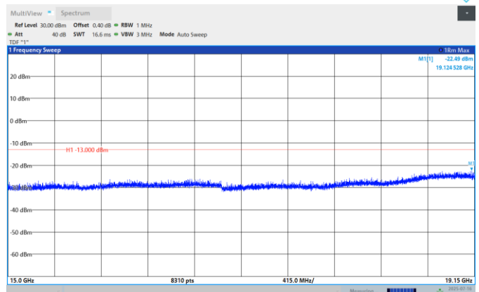
Band25-3MHz-QPSK-26340-1RB#0- Range:15000MHz~19150MHz
