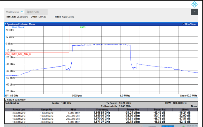
Band25-20MHz-QPSK-26590-100RB#0
