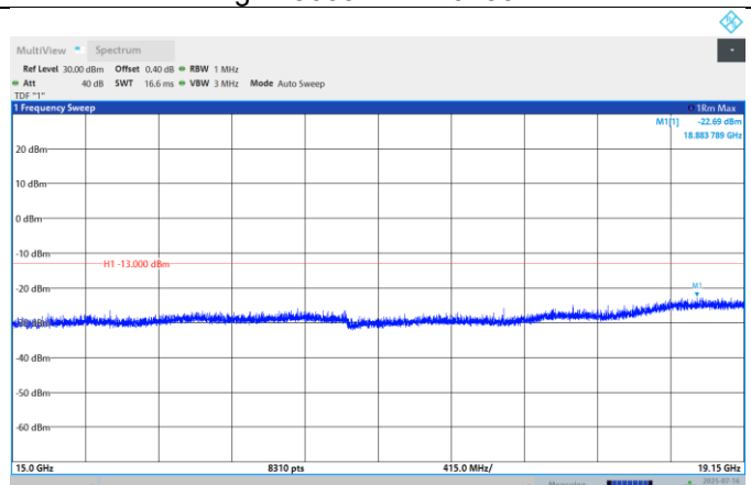
Band25-20MHz-QPSK-26590-1RB#0-Range:15000MHz~19150MHz
