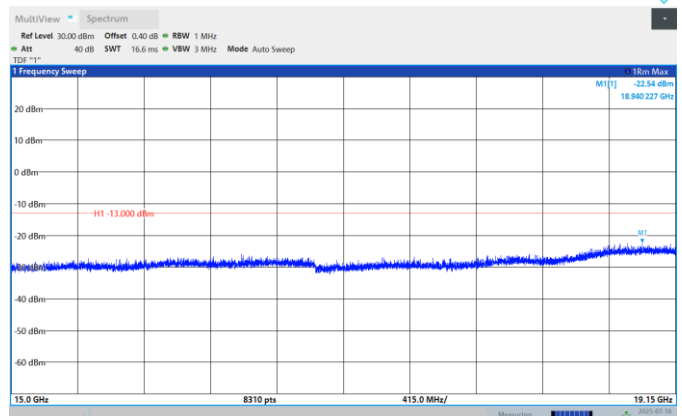
Band25-20MHz-QPSK-26340-1RB#0-Range:15000MHz~19150MHz
