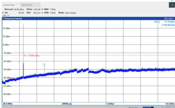
Band25-20MHz-QPSK-26340-1RB#0-Range:30~15000MHz
