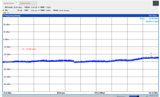
Band25-1.4MHz-QPSK-26340-1RB#0- Range:15000MHz~19150MHz
