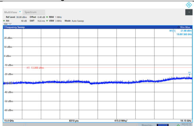
Band25-20MHz-QPSK-26590-1RB#0-Range:15000MHz~19150MHz
