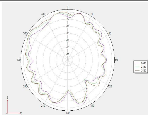
WIF/BT: 2410Mhz
