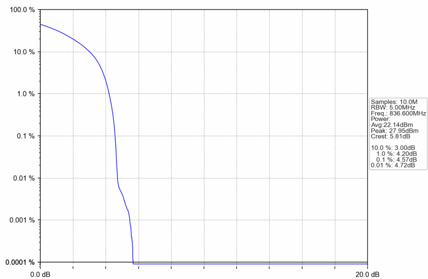
Band5_HSUPA_MCH_836.6MHz_Subtest 1_NTNV
