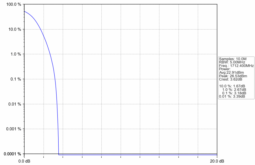
Band4_HSUPA_LCH_1712.4MHz_Subtest 1_NTNV
