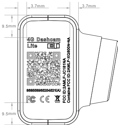
镭雕线框图
