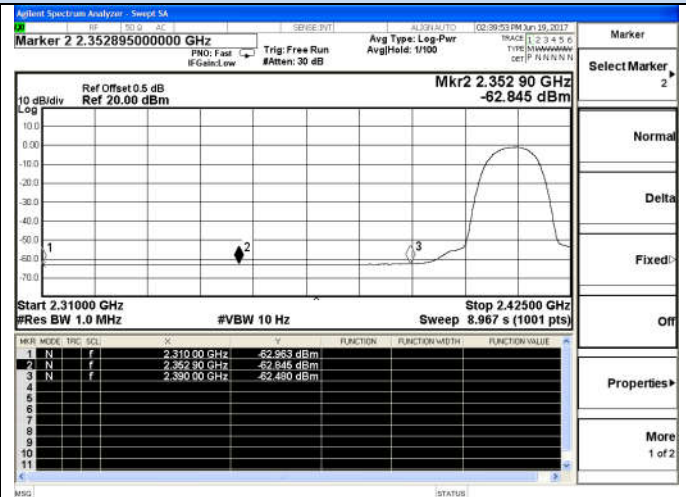
802.11b-Low channel(Average)
