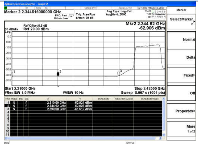
802.11n(HT20)-Low channel(Average)
