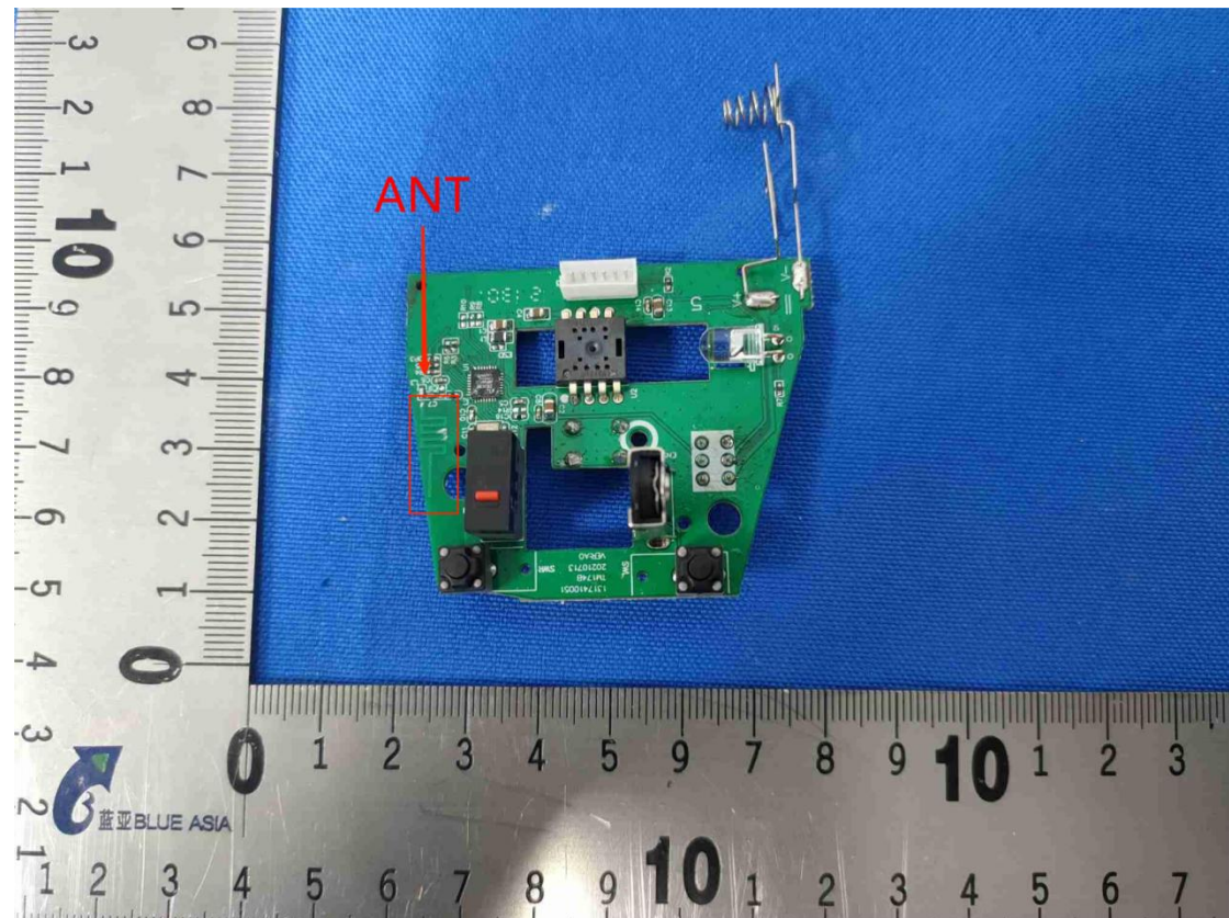
EUT Antenna
