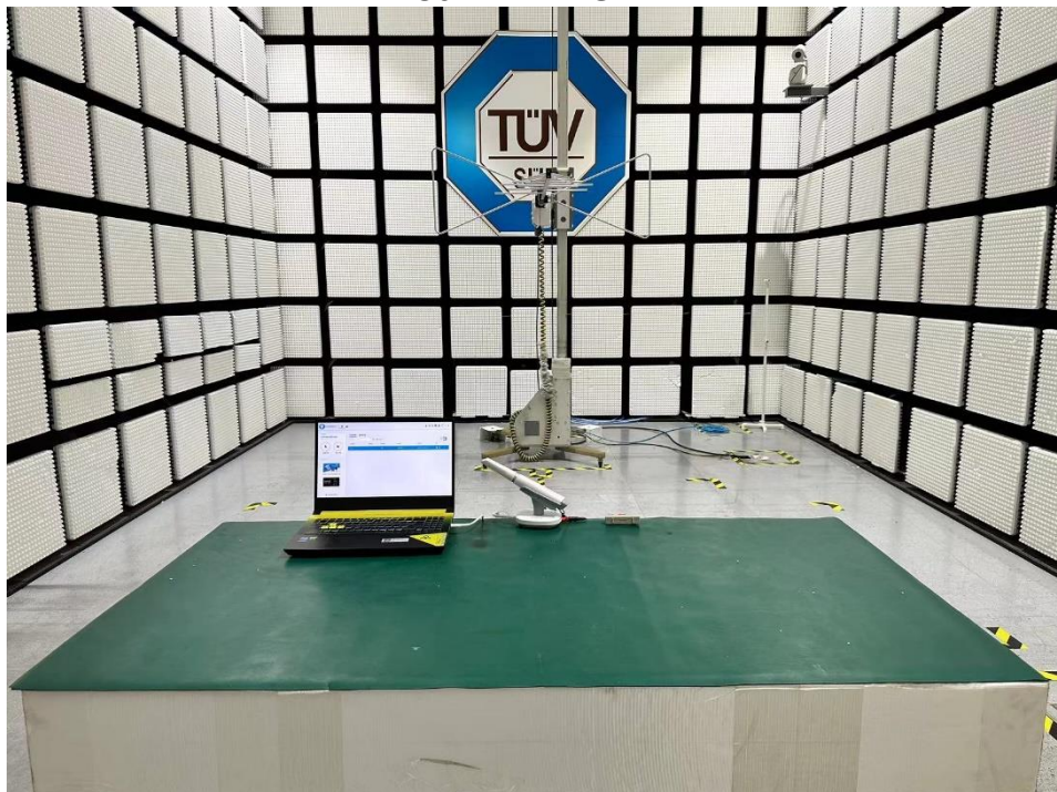
30MHz ~ 1GHz
