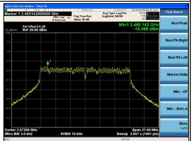
PSD - CH 13 - 802.11g
