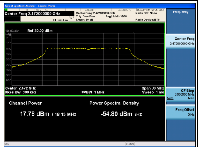
802.11g - AV Output power - CH 13
