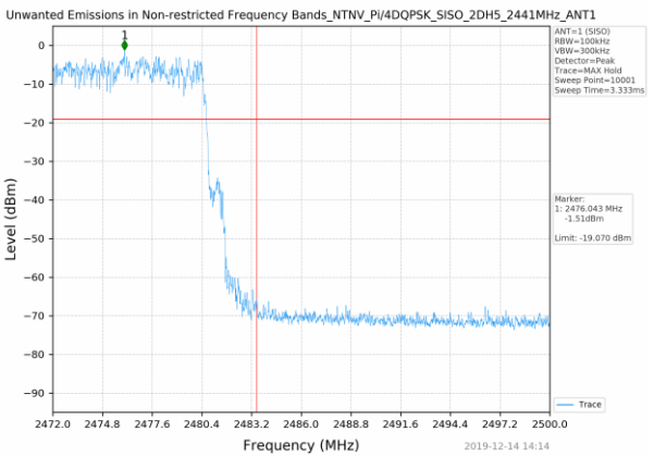
Right Band edge hopping on
