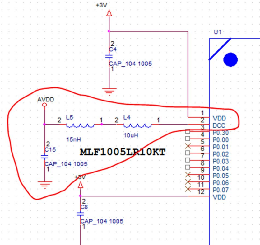
REV11 after → C15, L5, L4 소자 추가
