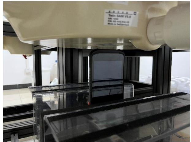
Bottom Side
