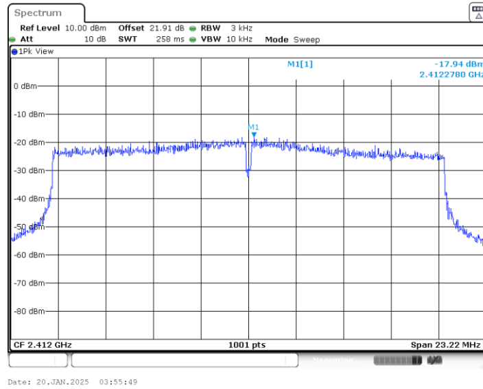
11AX20MIMO_Ant4_2412
