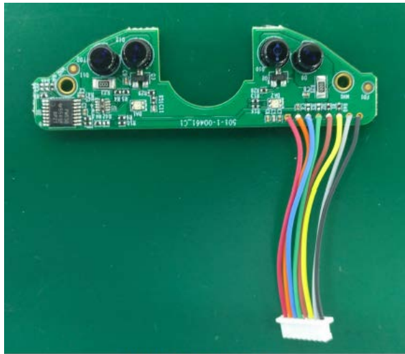
ALS PCB Top View
