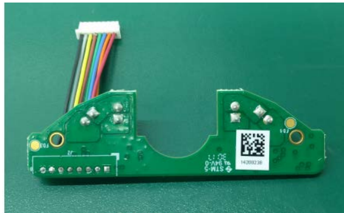
ALS PCB Bottom View
